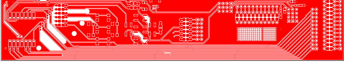
Top Layer (Scale 1:1.43)
